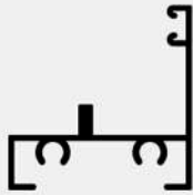
BI.FOLD DOOR OUTER TOP (BFD-01)
