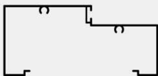
SHOPFRONT 4" (SPEK ALX) DOOR JAMB
